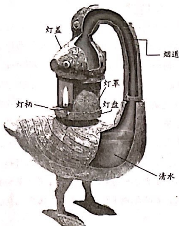
图1 汉代彩绘雁鱼青铜灯结构示意图
