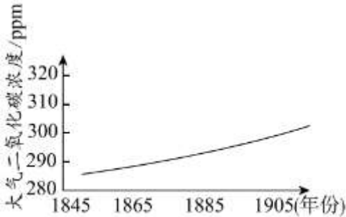
大气二氧化碳浓度变化曲线图
