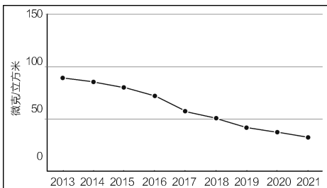
图1 2013-2021年北京市空气中PM2.5年平均浓度值变化趋势图
