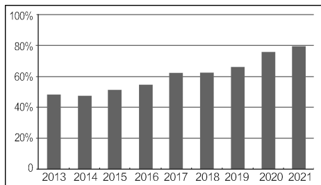
图2 2013-2021年北京市空气质量达标天数统计图
