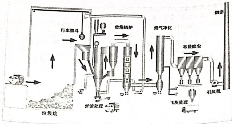
垃圾焚烧工艺流程图
