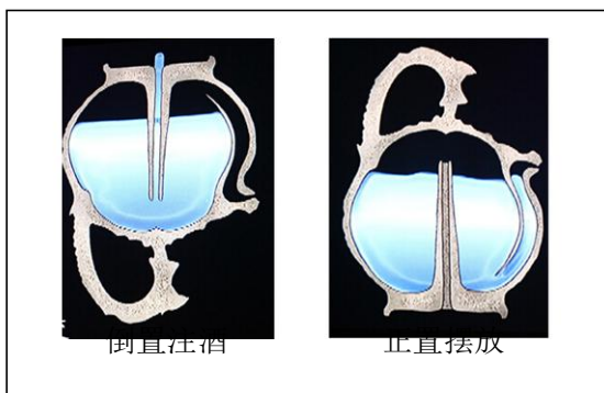
青釉提梁倒注壶原理示意图
