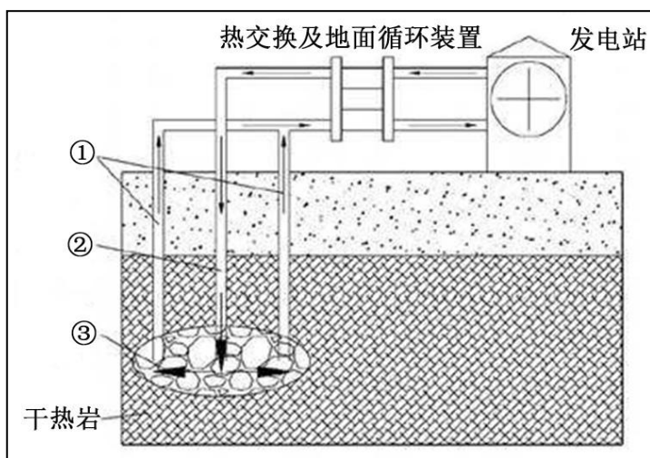
干热岩发电示意图
