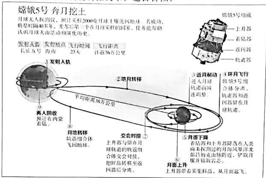
图1 嫦娥5号奔月挖土
