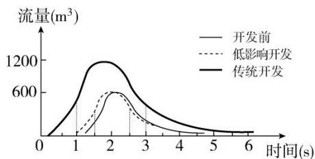
低影响开发与传统开发水文 ② 比较示意图
