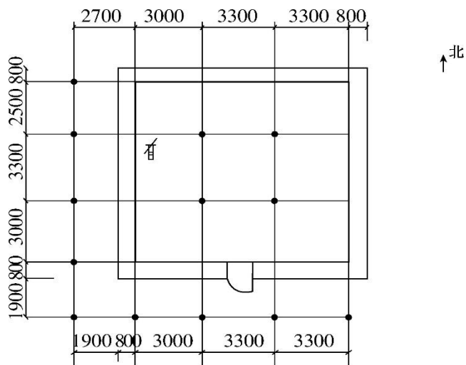
主体外设“L”形架空柱网平面图（单位 mm）
