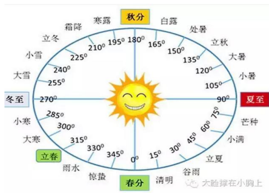
根据太阳位置划分的 24 节气图
