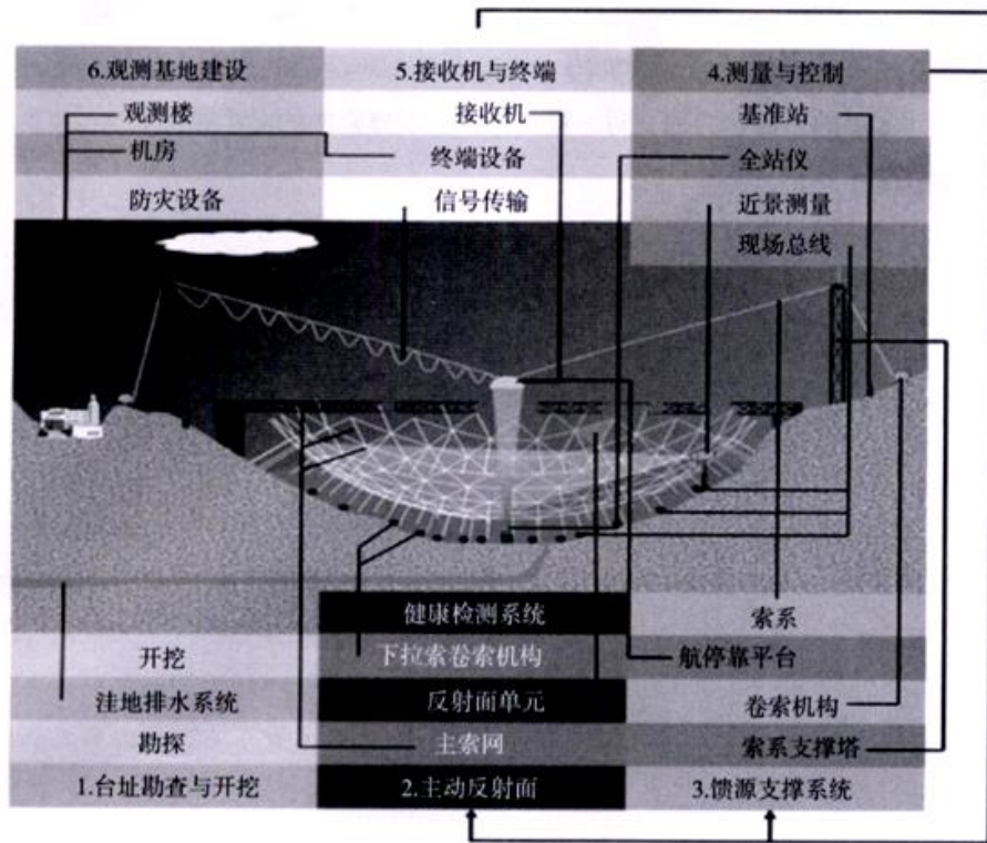
图一 FAST 天眼的系统构成
