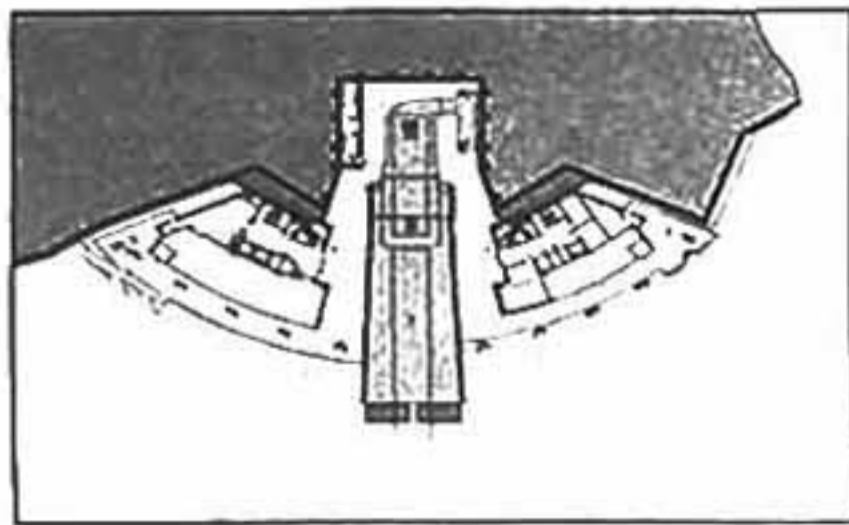
高山滑雪中心山顶出发区平面图
