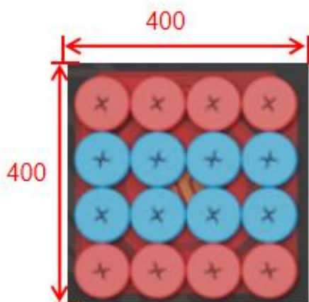
图 4.2-21 红方圆饼摆放示意图（俯视图）
