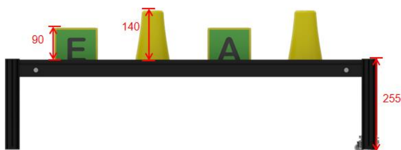
图 4.2-9 可移动资源岛示意图（正视图）
