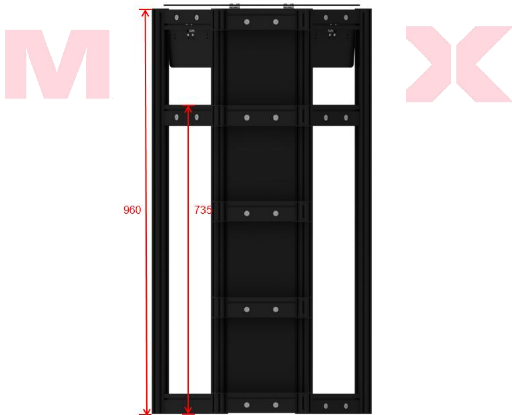
图 4.2-14 中央熔炉示意图（正视图）
